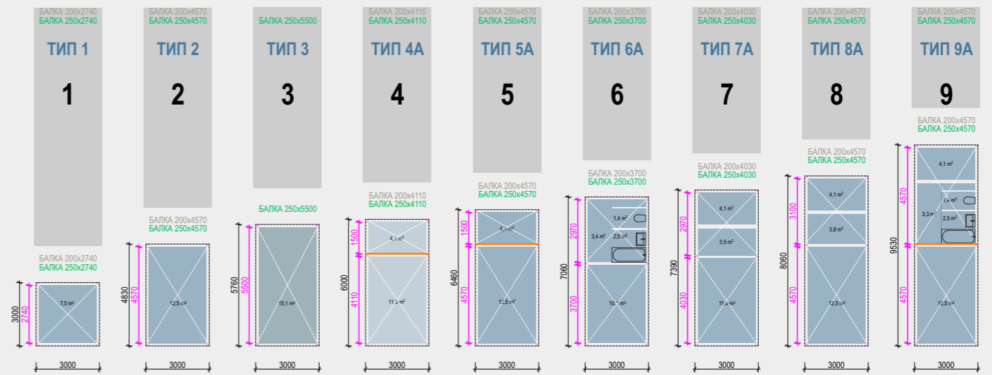
T - 4 Коридорные модули T - 4 Corridor module
